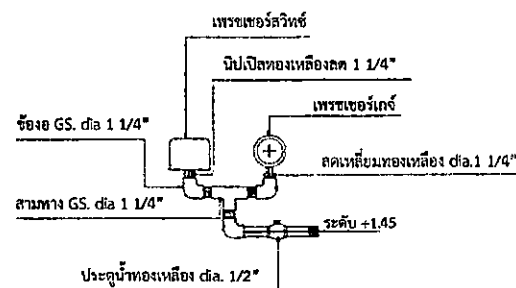
แบบขยายสิทธิควบคุมและแบ่งวัดความดัน no scale
